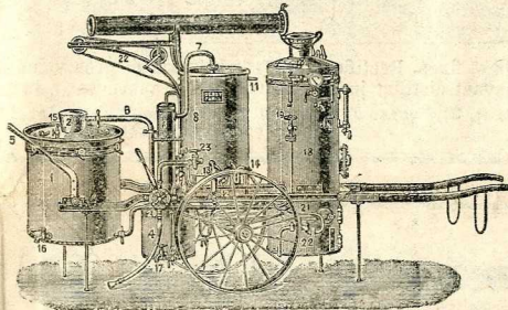
Fig. 186. — Alembic à vapeur sur chariot à distillation rapide
