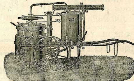
Fig. 65 bis. — Alembic sur chariot Produit sans repasse, de l'eau-de-vie rectifiée avec une économie considérable d'eau de temps et de combustible (On peut aussi, à volonté, opérer par repasse)
