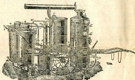
Fig. 185. — Appareil à 2 vases basculants
