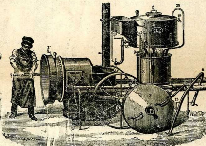
Fig. 99. — Alembic brûleur avec chauffe-vin Système Dero, breveté s.g.d.g. sur chariot en fer
