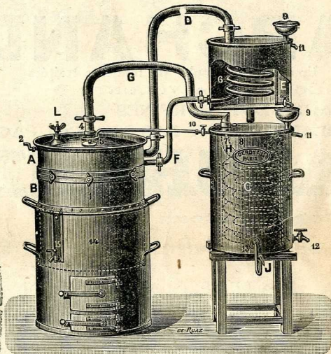
Fig. 204 bis. — Nouvel alembic Dero breveté s.g.d.g. avec chapiteau à repasse immédiate s'opérant séparément bien qu'en même temps que la distillation
