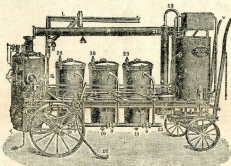
Fig. 176. — Appareil à vapeur à 3 ou 4 vases pour la distillation des Marcs, Fruits, Lies, Mûts épais, Vins, Cidres, etc. Appareil robuste construit spécialement pour les distillateurs ambulants
