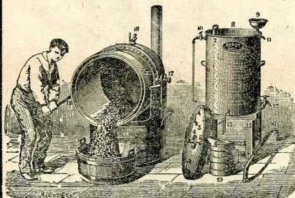
Fig. 76. — Alembic Dero avec système de basculement A partir de 300 litres, nous appliquons le basculement à cames (comme dans fig. 99)
